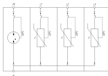
Схема электрическая принципиальная УЗИТ серии ГРОЗОСТОП® ГСКЗ-230/10 3+1
