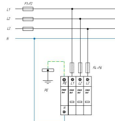
Схема подключения УЗИТ серии ГРОЗОСТОП® ГСКЗ-230/10 3+1 для сетей с системой заземления типа TT
