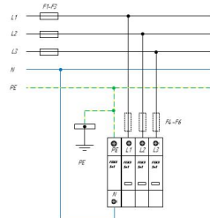
Схема подключения УЗИТ серии ГРОЗОСТОП® ГСКЗ-230/10 3+1 для сетей с системой заземления типа TN-S
