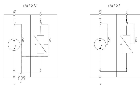
Схема электрическая принципиальная УЗМТ серии ГР030СТ0П® ГСКЗ-230/** 1+1 (C)
