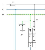
Схема подключения УЗМТ серии ГР030СТ0П® ГСКЗ-230/** 1+1 для сетей с системой заземления типа TN-S
