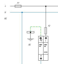
Схема подключения УЗМТ серии ГР030СТ0П® ГСКЗ-230/** 1+1 для сетей с системой заземления типа TT
