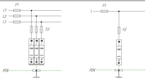
Схема подключения ГСВ3-230/10 для сети с системой заземления типа TN-C
