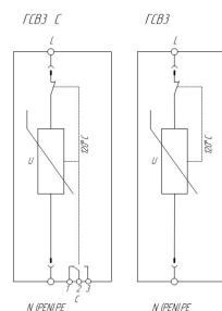
Схемы электрические принципиальные УЗВИ серии ГР030С100® ГСВ3 (C)
