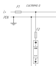
Схема подключения ГСВ3-230/10 для сети постоянного тока типа TN-C
