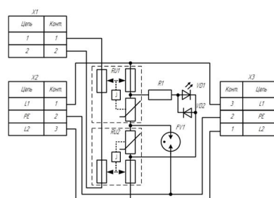
Схема электрическая принципиальная 53ИТ серии ГР030СТ01 ГСД3-230/IT
