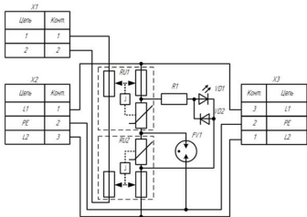
Схема электрическая принципиальная ГСДЗ-230/ІТ
