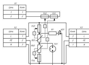
Схема электрическая принципиальная ГСДЗ-24, ГСДЗ-60, ГСДЗ-100
