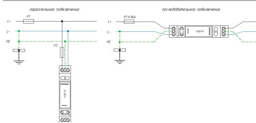
Схема подключения УЗИП ГСД3-24, 60, 100 для сетей постоянного тока типа TN-S система а
