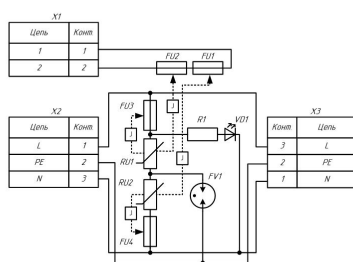
Схема электрическая принципиальная ГСД3-24, ГСД3-60, ГСД3-100
