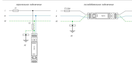
Схема подключения УЗИП ГСД3-24, 60, 100 для сетей переменного тока с системой заземления типа TN-S
