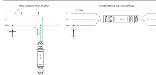
Схема подключения УЗИП ГСД3-24, 60, 100 для сетей постоянного тока типа TN-C система б
