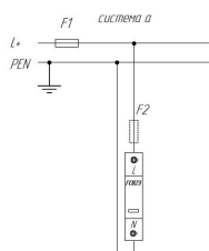
Схема подключения ГРЗОСТОП® ГСВ23-230/20 для сети постоянного тока типа TN-C
