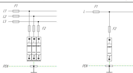
Схема подключения ГРЗОСТОП® ГСВ23-230/20 для сети с системой заземления типа TN-C
