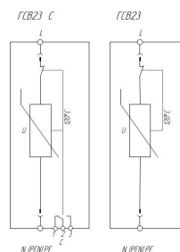
Схемы электрические принципиальные УЗИП серии ГРЗОСТОП® ГСВ23 (С)
