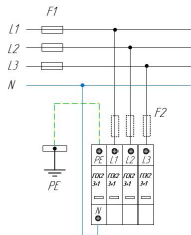
Схема подключения ГСК2 3+1 (С) для сетей с системой заземления типа TT
