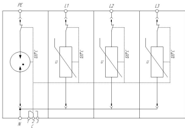
Схема электрическая принципиальная УЭИП серии ГРЗОДОТОП® ГСК2 3+1 С
