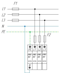
Схема подключения ГСК2 3+1 (С) для сетей с системой заземления типа TN-S
