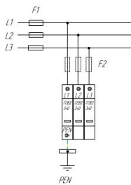
Схема подключения ГСВ2 3+0 К1 для сетей с системой заземления типа TN-C
