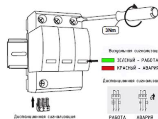
Визуальная и дистанционная сигнализация УЗИП серии ГСВ2 3+0 К1
