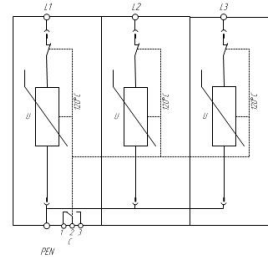
Схема электрическая принципиальная УЗИП серии ПРОЗДОСТОН® ГСВ2 3+0 С
