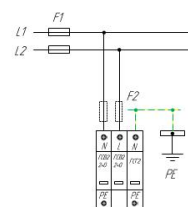
Схема подключения ГСВ2 2+0 (C), ГСВ2-230/20 для сети с системой заземления типа IT
