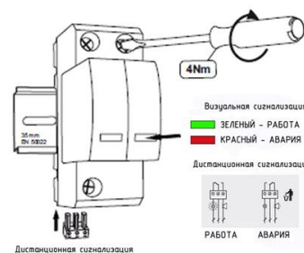
Визуальная и дистанционная сигнализация УЗМН серии ГСВ2 2+0 (C)
