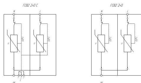
Схемы электрические принципиальные УЗМН серии ГРОЗДОСТОП® ГСВ2 2+0 (C)
