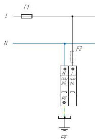
Схема подключения ГСВ2 2+0 (C) для сетей с системой заземления типа TN-S, TT
