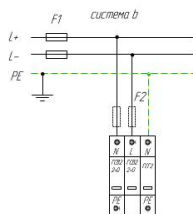
Схема подключения ГСВ2 2+0 (C), ГСВ2-230/20 для сети постоянного тока типа TN-S
