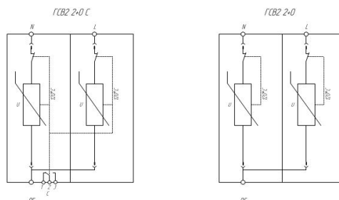
Схемы электрические принципиальные УЗИП серии ГРЗДОСТОП® ГСВ2 2+0 (C)
