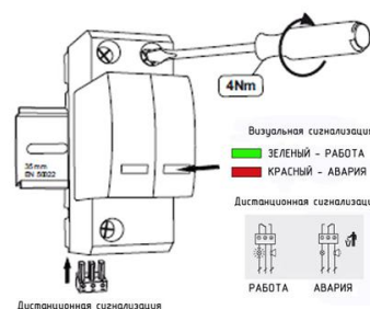
Визуальная и дистанционная сигнализация УЗИП серии ГСВ2 2+0 (C)
