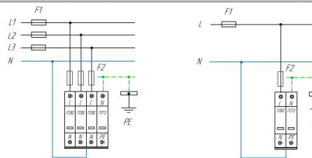
Схема подключения ГСВ2 (C) ГЛТ2-230/20 для сети с системой заземления типа TN-S
