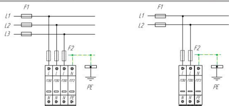
Схема подключения ГСВ2 (L) ГСВ2-230/20 для сети с системой заземления типа IT
