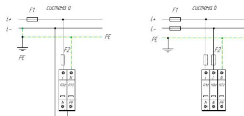
Схема подключения ГСВ2 (L) ГСВ2-230/20 для сети постоянного тока типа TN-S
