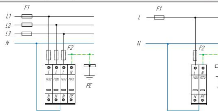
Схема подключения ГСВ2 (L) ГСВ2-230/20 для сети с системой заземления типа TT
