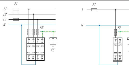
Схема подключения ГСВ2 (L) ГСВ2-230/20 для сети с системой заземления типа TN-S
