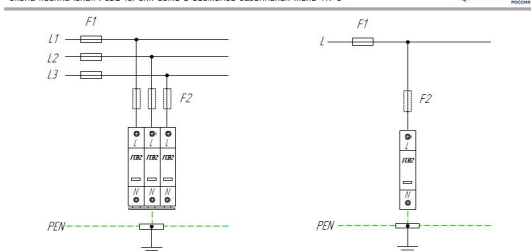
Схема подключения ГСВ2 IC1 для сети с системой заземления типа TN-C
