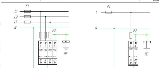
Схема подключения ГСВ2 IC1, ГСВ2-230/20 для сети с системой заземления типа TN-S
