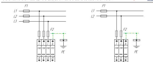
Схема подключения ГСВ2 IC1, ГСВ2-230/20 для сети с системой заземления типа IT
