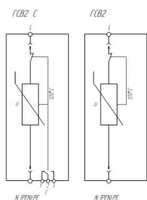
Схемы электрические принципиальные УЭИП серии ГР030С001® ГСВ2 IC1
