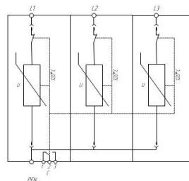
Схема электрическая принципиальная УЗИП серии ГРОЗДОСТОП® ГСВ2 3+0 С
