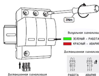
Визуальная и дистанционная сигнализация УЗИП серии ГСВ2 3+0 К1
