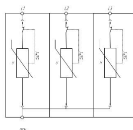
Схема электрическая принципиальная УЗМТ серии ГРОДОТОП® ГСВ2 3+0
