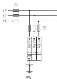
Схема подключения ГСВ2 3+0 (U) для сетей с системой заземления типа TN-C
