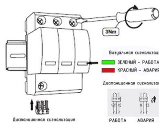
Визуальная и дистанционная сигнализация УЗИП серии ГСВ2 3+0 (U)
