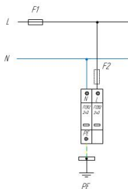
Схема подключения ГСВ2 2+0 (К) для сетей с системой заземления типа TN-S, TT
