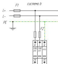
Схема подключения ГСВ2 2+0 (К), ГСВ2-230/20 для сети постоянного тока типа TN-S
