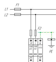
Схема подключения ГСВ2 2+0 (К), ГСВ2-230/20 для сети с системой заземления типа IT
