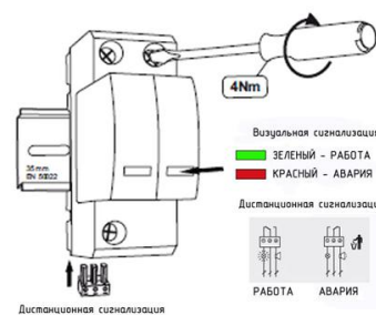
Визуальная и дистанционная сигнализация УЗИП серии ГСВ2 2+0 (К)
