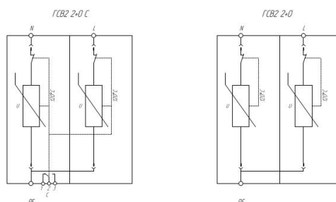
Схемы электрические принципиальные 53И1 серии ГРОЗДОТОН® ГСВ2 2+0 (С)
