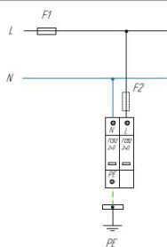
Схема подключения ГСВ2 2+0 (С) для сетей с системами заземления типа TN-S, TT
