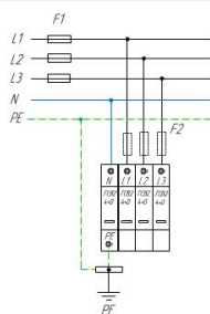
Схема подключения ГСВ2 4+0 (U) для сетей с системой заземления типа TN-S
