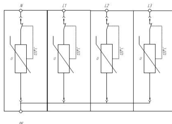
Схема электрическая принципиальная УЗИП серии ГРОЗДОСТОП® ГСВ2 4+0
