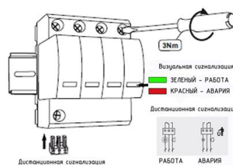
Визуальная и дистанционная сигнализация УЗИП серии ГСВ2 4+0 (U)
