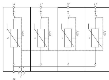
Схема электрическая принципиальная УЗИП серии ПРОЗДОТОН® ГСВ2 4+0 С
