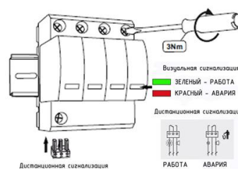
Визуальная и дистанционная сигнализация УЗИП серии ГСВ2 4+0 К)
