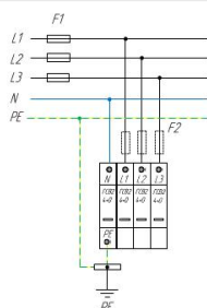
Схема подключения ГСВ2 4+0 К) для сетей с системой заземления типа TN-S
