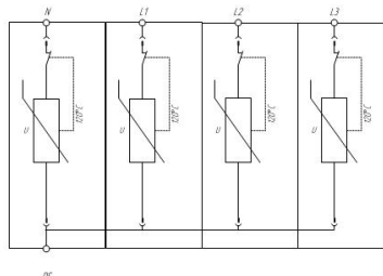
Схема электрическая принципиальная УЗИП серии /ПРОДОЛЖЕНИЕ/ ГСВ2 4+0
