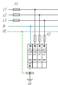
Схема подключения ГСВ2 4+0 (C) для сетей с системой заземления типа TN-S
