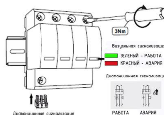
Визуальная и дистанционная сигнализация УЗИП серии ГСВ2 4+0 (C)
