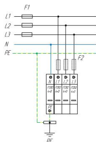
Схема подключения ГСВ2 4+0 (С) для сетей с системой заземления типа TN-S
