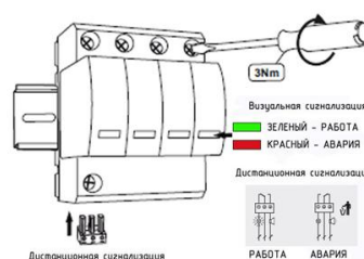
Визуальная и дистанционная сигнализация УЗИП серии ГСВ2 4+0 (С)
