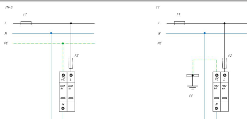
Схема подключения ГСК2 1+1 (C) для сетей с системой заземления типа TN-S, TT
