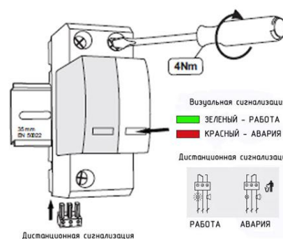
Визуальная и дистанционная сигнализация УЗИП серии ГСК2 1+1 (C)
