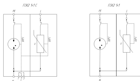
Схемы электрические принципиальные УЗИП серии ГРОЗОСТОП® ГСК2 1+1 (C)
