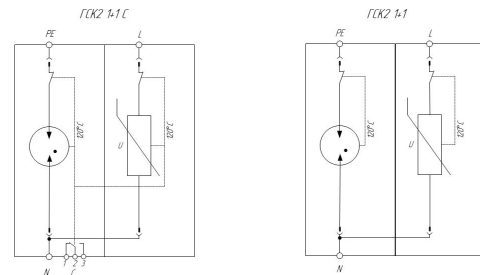
Схемы электрические принципиальные УЗИП серии ГРОЗОСТОП® ГСК2 1+1 (К)
