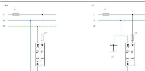
Схема подключения ГСК2 1+1 (К) для сетей с системой заземления типа TN-S, TT
