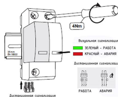
Визуальная и дистанционная сигнализация УЗИП серии ГСК2 1+1 (К)
