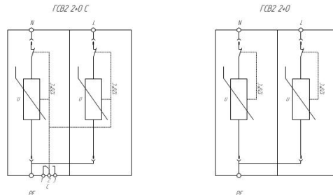
Схемы электрические принципиальные УЗИП серии ГРЗДОСТОП® ГСВ2 2+0 (К)
