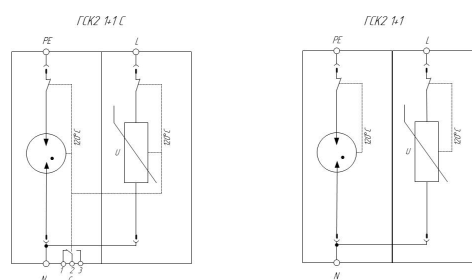
Схемы электрические принципиальные УЗМТ серии ГР030СТ01® ГСК2 1+1 (C)
