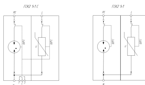
Схемы электрические принципиальные УЗиПТ серии ГР030СТ01® ГСК2 1+1 (К)
