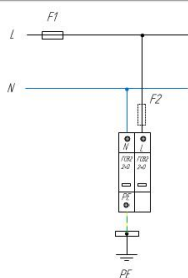
Схема подключения ГСВ2 2+0 (С) для сетей с системой заземления типа TN-S, TT
