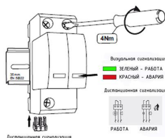
Визуальная и дистанционная сигнализация УЗМН серии ГСВ2 2+0 (С)
