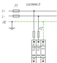
Схема подключения ГСВ2 2+0 (С), ГСВ2-230/20 для сети постоянного тока типа TN-S
