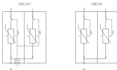
Схемы электрические принципиальные УЗМН серии ГРЗВСТ017® ГСВ2 2+0 (С)
