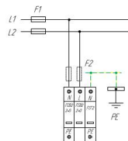
Схема подключения ГСВ2 2+0 (С), ГСВ2-230/20 для сети с системой заземления типа IT
