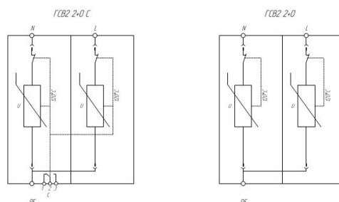
Схемы электрические принципиальные УЗМП серии ПРОДОЛЖИТЕЛЬ ГСВ2 2+0 (С)
