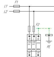
Схема подключения ГСВ2 2+0 (С), ГСВ2-230/20 для сети с системой заземления типа IT
