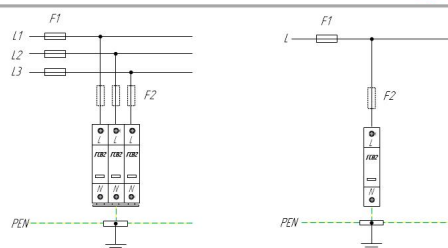
Схема подключения ГСВ2 (C) для сети с системой заземления типа TN-C
