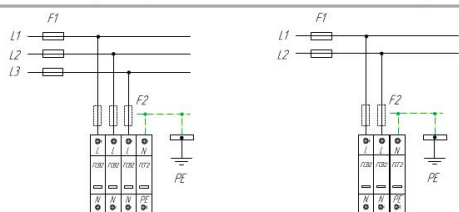
Схема подключения ГСВ2 (C) ГТ2-230/20 для сети с системой заземления типа IT
