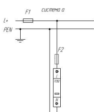
Схема подключения ГСВ2 (C) для сети постоянного тока типа TN-C
