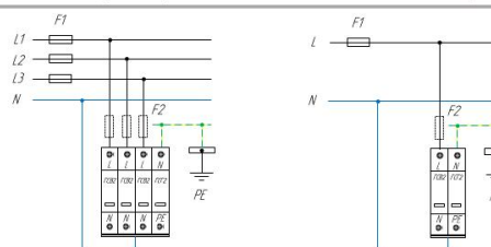
Схема подключения ГСВ2 (C) ГТ2-230/20 для сети с системой заземления типа TN-S
