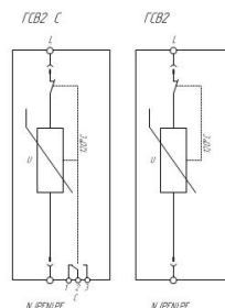
Схемы электрические принципиальные УЗИП серии ГРОЗДОСТОП® ГСВ2 (C)
