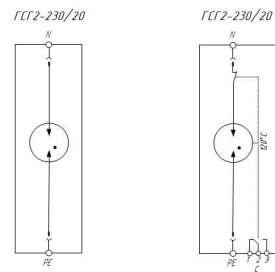
Схемы электрические принципиальные УЗИП серии ГРОЗДОСТОП® ГСГ2-230/20 (С)
