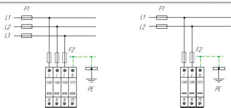
Схема подключения ГСБ2 (С), ГСГ2-230/20 для сети с системой заземления типа IT
