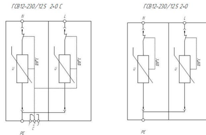
Схема электрическая принципиальная УЗИП серии ГР030С107® ГСВ12-230/12,5 2+0 (К)
