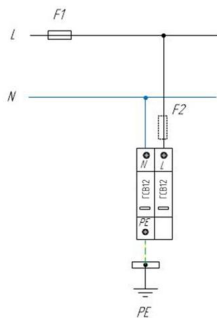
Схема подключения ГСВ12-230/12,5 2+0 (К) для сетей с системой заземления типа TN-S
