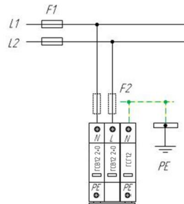
Схема подключения ГСВ12-230/12,5 2+0 (К) для сетей с системой заземления типа TT
