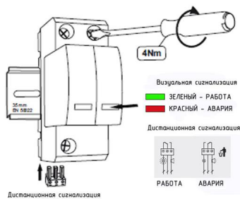
Визуальная и дистанционная сигнализация УЗИП серии ГСВ12-0 (К)
