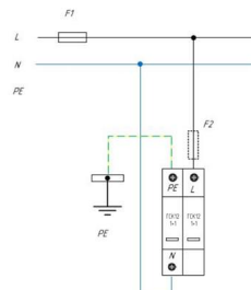
Схема подключения ГСК12-230/12,5 1+1 (С) для сетей с системой заземления типа TT
