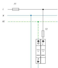
Схема подключения ГСК12-230/12,5 1+1 (С) для сетей с системой заземления типа TN-S
