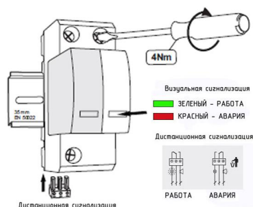
Визуальная и дистанционная сигнализация УЗИП серии ГСК1 1+1 (С)
