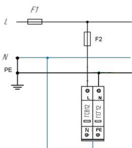
Схема подключения ГСВ12-230/12,5 (C) для сетей с системой заземления типа TN-S
