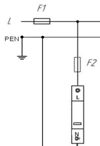
Схема подключения ГСВ12-230/12,5 (C) для сетей с системой заземления типа TN-C
