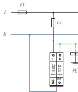
Схема подключения ГСВ12-230/12,5 (C) для сетей с системой заземления типа TT
