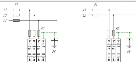
Схема подключения ГСВ1 1-0 (C), ГСГ1 для сети с системой заземления типа IT
