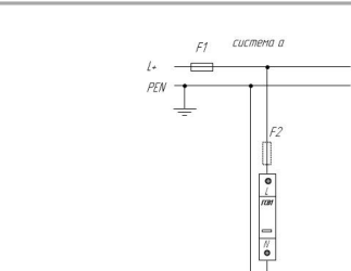
Схема подключения ГСВ1 (C) для сети постоянного тока типа TN-C
