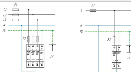
Схема подключения ГСВ1 1-0 (C), ГСГ1 для сети с системой заземления типа TN-S
