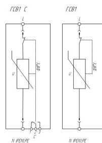
Схемы электрические принципиальные УСМП серии ГРОЗДОСТОЙ® ГСВ1 (C)
