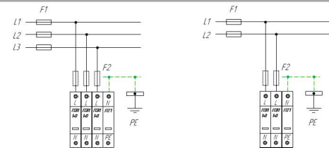
Схема подключения ГСВ1 1-0 (C), ГСГ1 для сети с системой заземления типа IT
