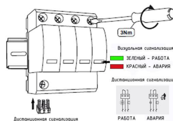
Визуальная и дистанционная сигнализация УЗИП серии ГСВ1 4+0 (Г)
