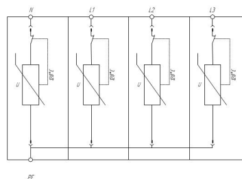
Схема электрическая принципиальная УЗВИ серии ПРОДОСТОП® ГСВ1 4+0
