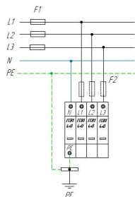
Схема подключения ГСВ1 4+0 (Г) для сетей с системой заземления типа TN-S
