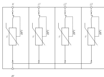
Схема электрическая принципиальная УЗВИП серии ГРОЗДОСТОП® ГСВ1 4+0
