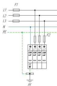
Схема подключения ГСВ1 4+0 (С) для сетей с системой заземления типа TN-S
