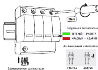
Визуальная и дистанционная сигнализация УЗИП серии ГСВ1 4+0 (С)
