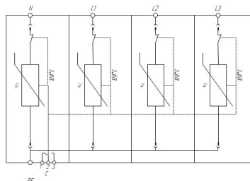
Схема электрическая принципиальная УЗИП серии ГРОЗДОСТОП® ГСВ1 4+0 С
