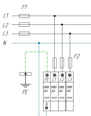
Схема подключения ГСК1 3+1 (С) для сетей с системой заземления типа TT
