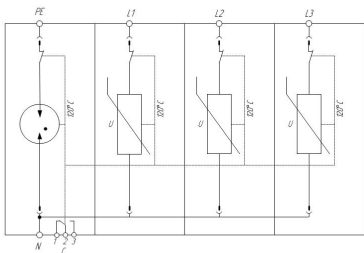
Схема электрическая принципиальная УЗМ1 серии ГРОЗОСТОП® ГСК1 3+1 С
