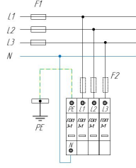
Схема подключения ГСК1 3+1 (С) для сетей с системой заземления типа TT
