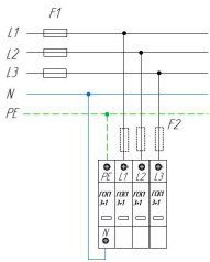
Схема подключения ГСК1 3+1 (С) для сетей с системой заземления типа TN-S
