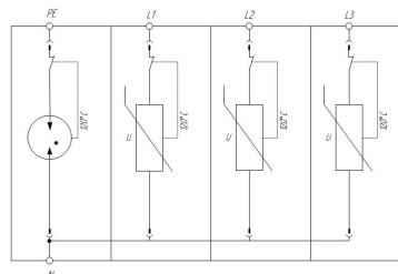
Схема электрическая принципиальная УЗИП серии ПРОДОСТОП® ГСК1 3+1
