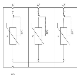
Схема электрическая принципиальная УЗИП серии ГРОЗДОСТОП® ГСВ1 3-0
