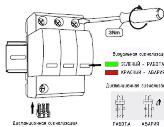
Визуальная и дистанционная сигнализация УЗИП серии ГСВ1 3+0 (C)
