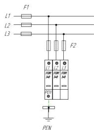
Схема подключения ГСВ1 3+0 (C) для сетей с системой заземления типа TN-C
