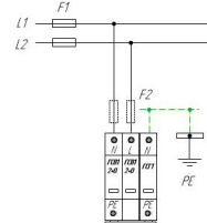
Схема подключения ГСВ1 2+0 (C) ГСГ1-230/25 для сети с системой заземления типа IT
