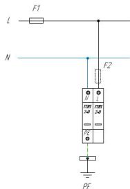
Схема подключения ГСВ1 2+0 (C) для сетей с системой заземления типа TN-S, TT
