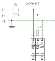
Схема подключения ГСВ1 2+0 (C) ГСГ1-230/25 для сети постоянного тока типа TN-S
