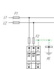
Схема подключения ГСВ1 2+0 (C) ГСГ1-230/25 для сети с системой заземления типа IT
