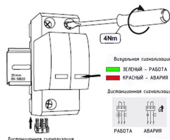
Визуальная и дистанционная сигнализация УЗИП серии ГСВ1 2+0 (C)
