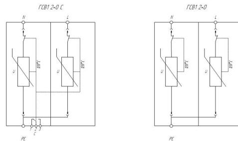
Схемы электрические принципиальные УЗМП серии ГР030С001® ГСВ1 2-0 (C)
