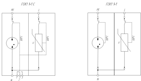
Схемы электрические принципиальные УЗМ1 серии ГР030СТ01® ГСК1 1+1 (С)
