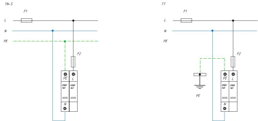
Схема подключения ГСК1 1+1 (С) для сетей с системой заземления типа TN-S, TT
