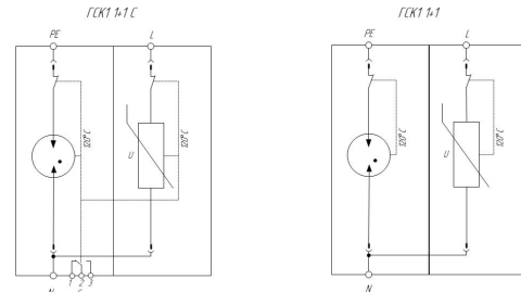
Схемы электрические принципиальные УЗИП серии ГРОЗОСТОП® ГСК1 1+1 (C)
