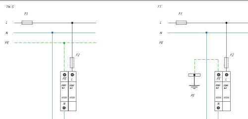
Схема подключения ГСК1 1+1 (C) для сетей с системой заземления типа TN-S, TT
