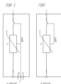
Схемы электрические принципиальные УЗМТ серии ГРОЗДОСТОН® ГСВ1 (C)
