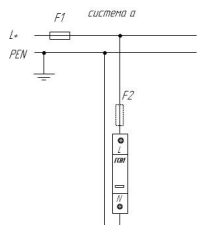
Схема подключения ГСВ1 (C) для сети постоянного тока типа TN-C
