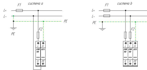
Схема подключения ГСВ1 1-0 (C), ГСВ1 для сети постоянного тока типа TN-S
