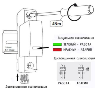
Визуальная и дистанционная сигнализация УЗИП серии ГСВ1 (C)
